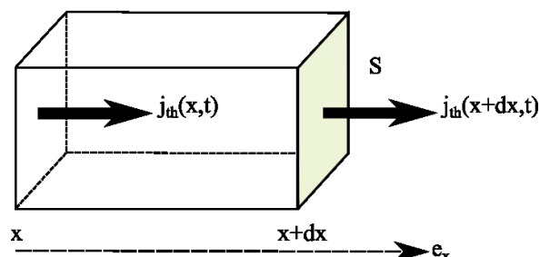
Figure 16 - Représentation d'un élément élémentaire de longueur dx
