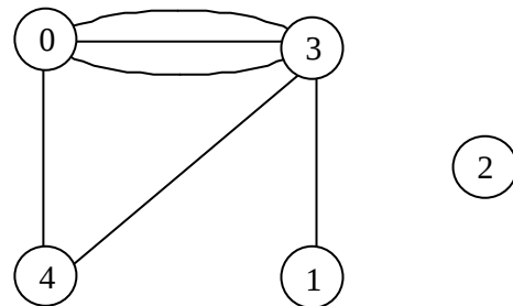
Le graphe G_{ex1}
