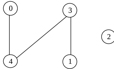
Le graphe H(G_{ex1})
