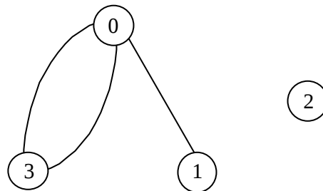
Le graphe K(G_{ex1})
