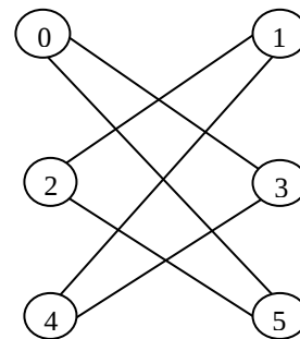
Le graphe Gex2
