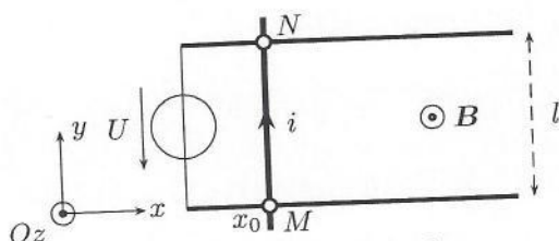
FIG. 2 - Rails de Laplace
