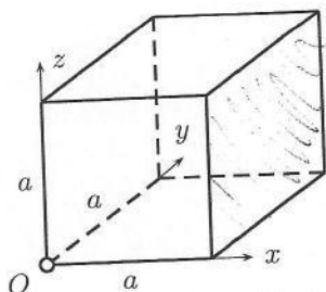
FIG. 1 - Boîte cubique d'arête a
