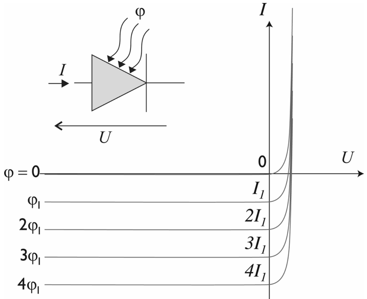
Figure 4 : Caractéristique de la photodiode
