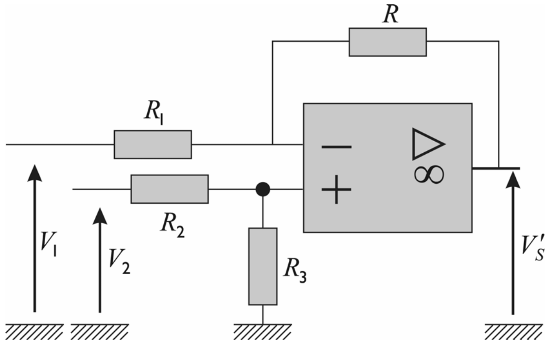
Figure 3 : montage soustracteur
