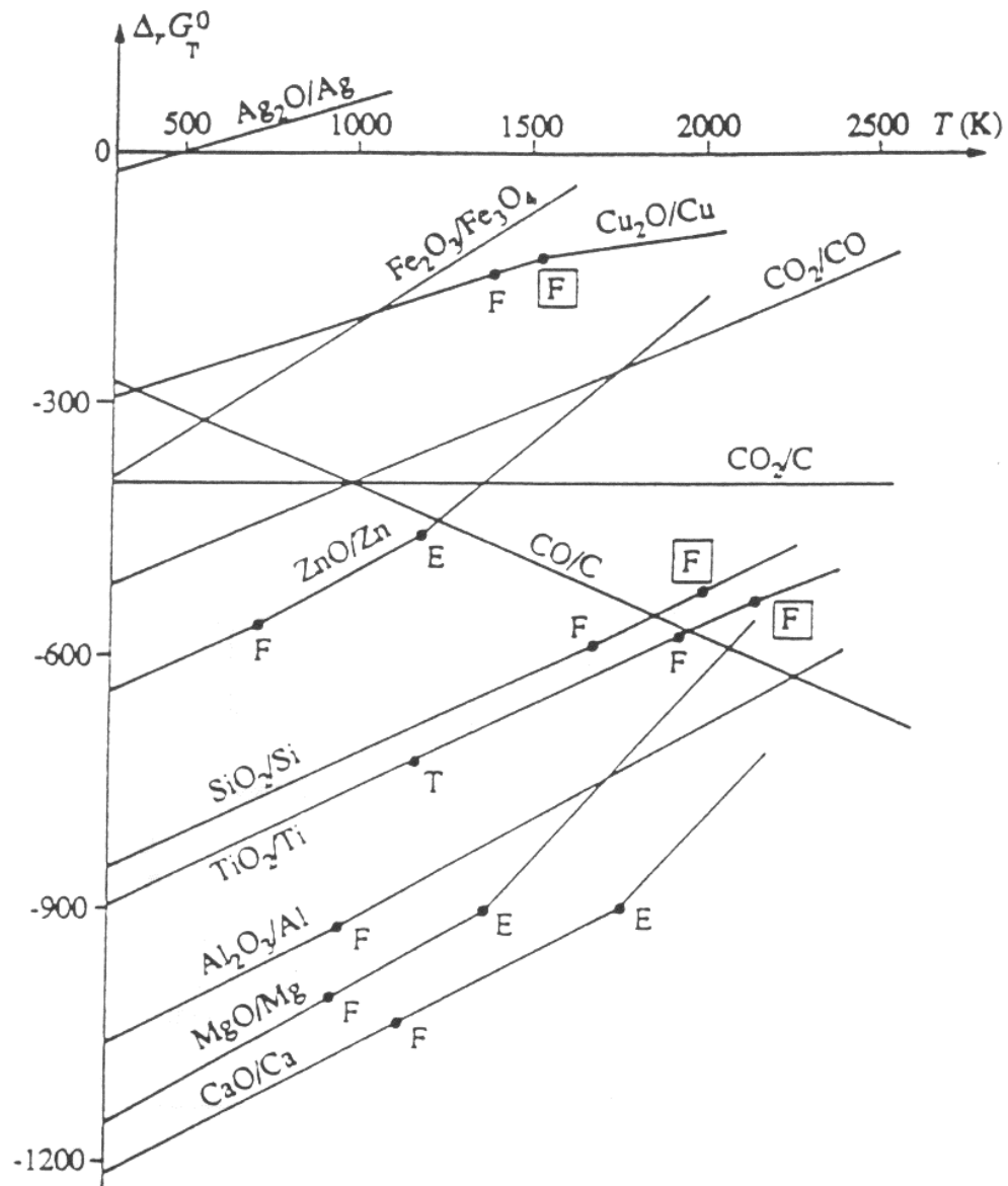
fig. 2: Diagramme d'Ellingham.
