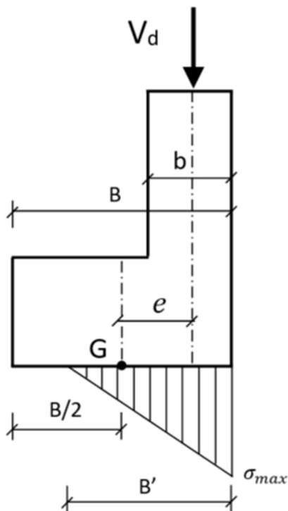
Figure 3 : répartition triangulaire des contraintes sous la semelle
