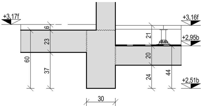
Détail n°1 à compléter
