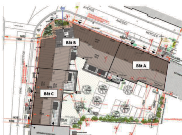
Figure 7 : plan de masse (sans échelle)
