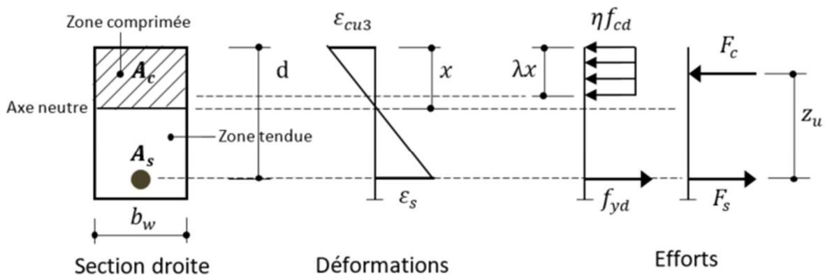
Figure 14 : diagramme rectangle simplifié
