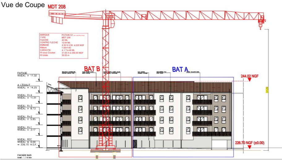
Sans échelle – coupe indicative
