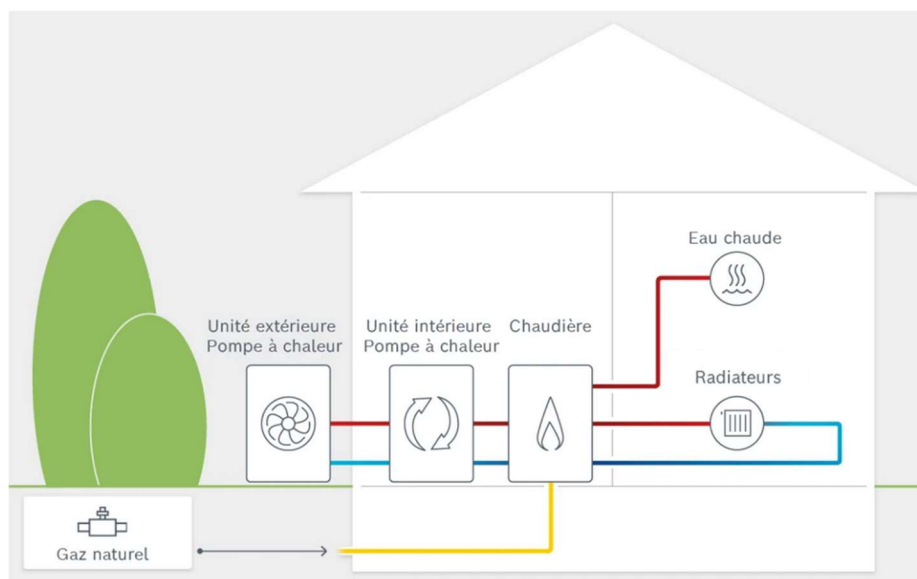
Figure 22 : schéma de principe d'un système hybride
