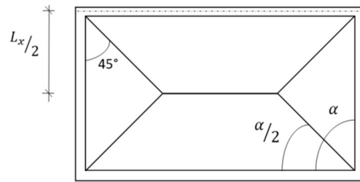
Figure 12 : dalle sur quatre côtés
