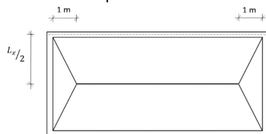
Figure 11 : dalle sur deux côtés
