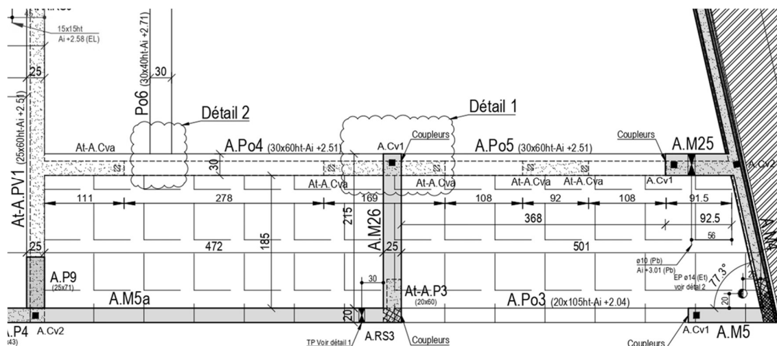
Figure 17 : poutre continue définitive réalisée (à deux travées)
