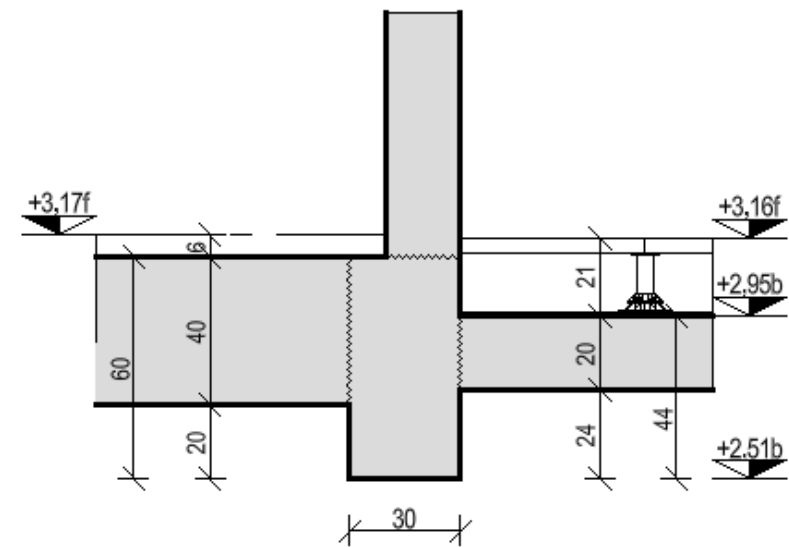
Détail n°2 à compléter
