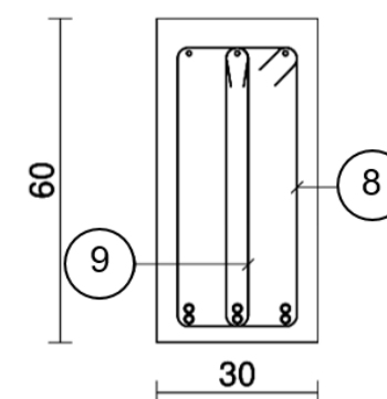
Coupe A-A (sans échelle)
