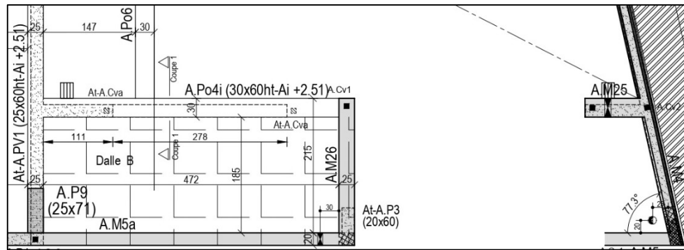
Figure 16 : poutre Po4i isostatique de la phase provisoire
