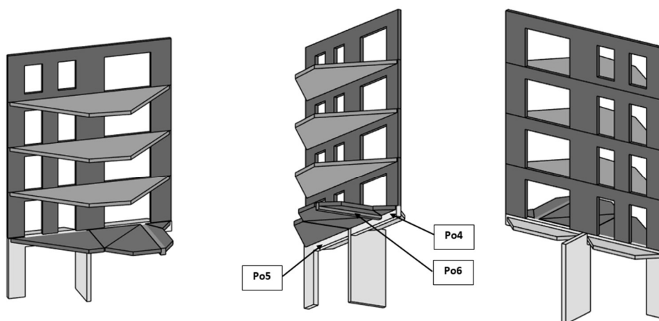
Figure 13 : extrait du modèle 3D revit - la charpente n'est pas représentée
