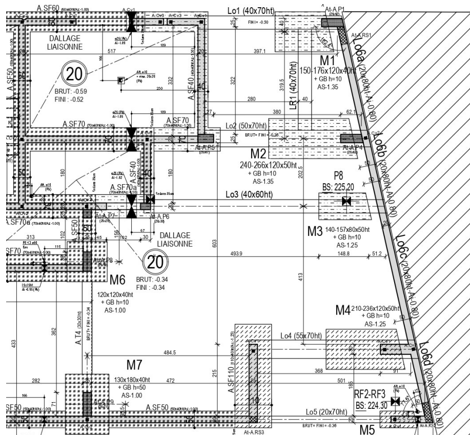
Figure 4 : plan de coffrage des fondations
